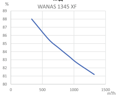
кпд
