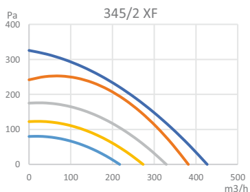
SPRAWNOŚĆ/WYDAJNOŚĆ
