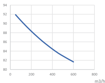
[%] SPRAWNOŚĆ/WYDAJNOŚĆ
