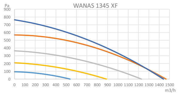
SPRĘŻ/WYDAJNOŚĆ
