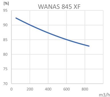
SPRAWNOŚĆ/WYDAJNOŚĆ
