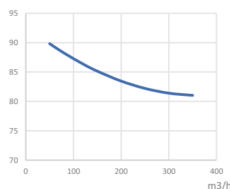
[%] SPRAWNOŚĆ/WYDAJNOŚĆ
