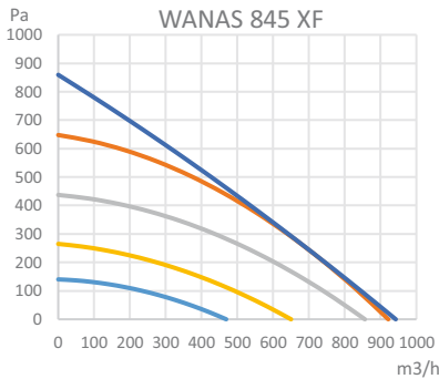
SPRĘŻ/WYDAJNOŚĆ
