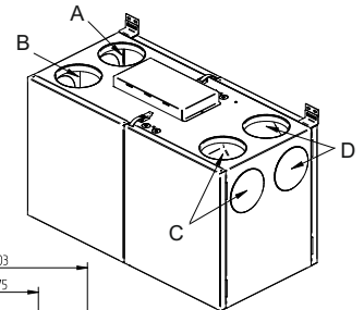
Konfiguracja prawa
