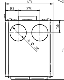
Konfiguracja prawa
