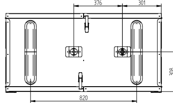
Konfiguracja prawa
