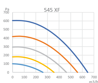
SPRAWNOŚĆ/WYDAJNOŚĆ
