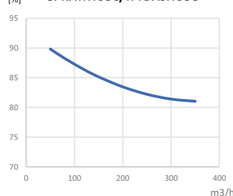
SPRAWNOŚĆ/WYDAJNOŚĆ
