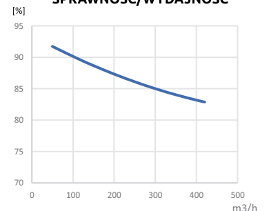
SPRĘŻ/WYDAJNOŚĆ
