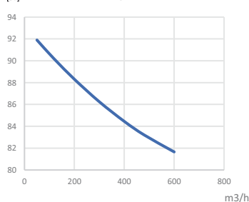
SPRAWNOŚĆ/WYDAJNOŚĆ
