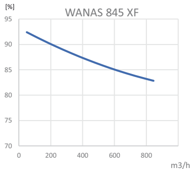
SPRAWNOŚĆ/WYDAJNOŚĆ
