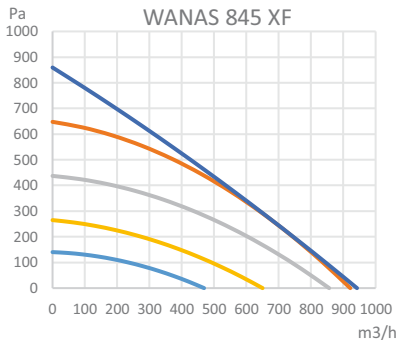
SPRĘŻ/WYDAJNOŚĆ
