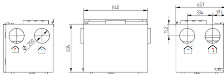
Wersja prawa
