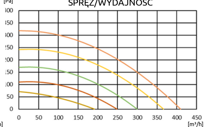
SPRĘŻ/WYDAJNOŚĆ
