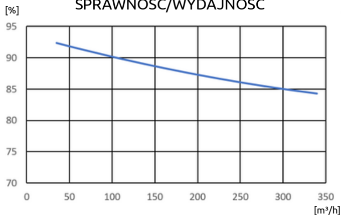
SPRAWNOŚĆ/WYDAJNOŚĆ
