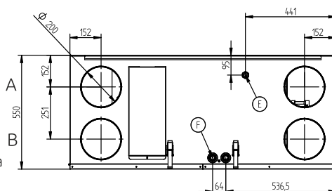
WERSJA LEWA
