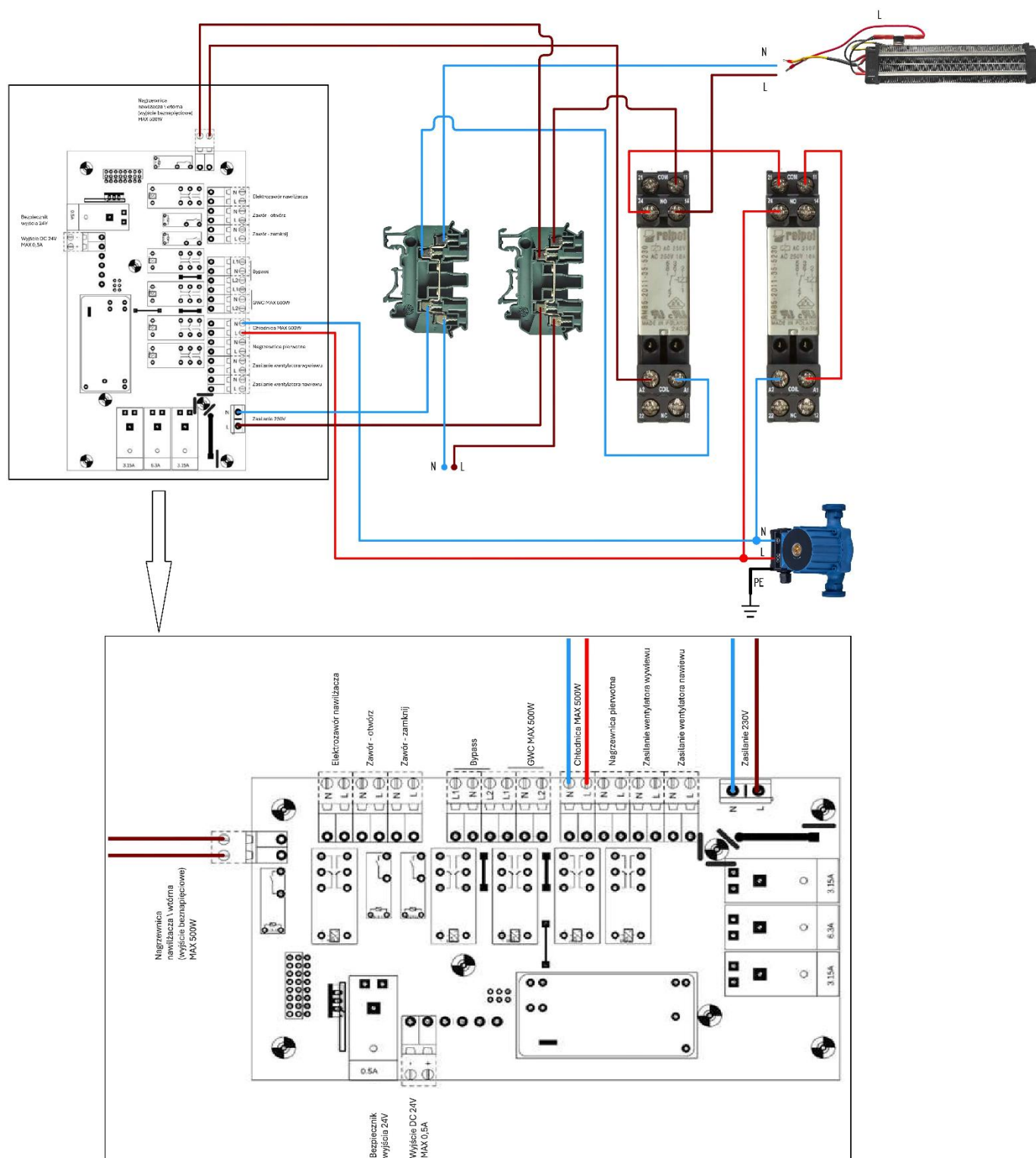
Schemat podłączenia pompy obiegowej do płyty głównej rekuperatora.
